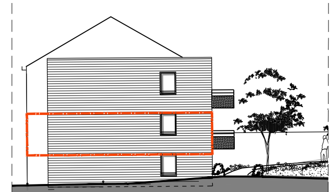
FACADE SUD-OUEST
