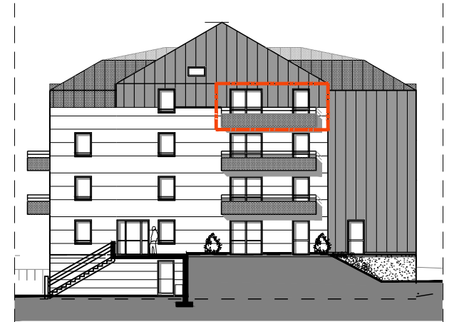
FACADE NORD-OUEST
