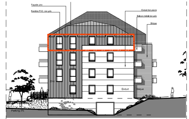
FACADE SUD-OUEST
