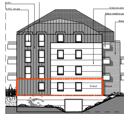
FACADE SUD-OUEST
