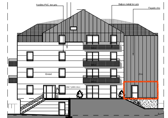
FACADE NORD-OUEST
